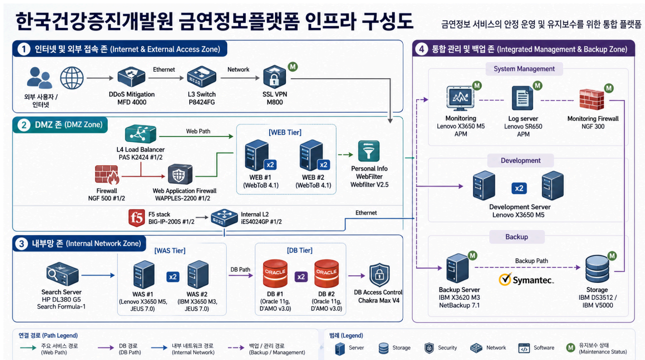
그림 1. 금연서비스 통합정보시스템 인프라 구성도
